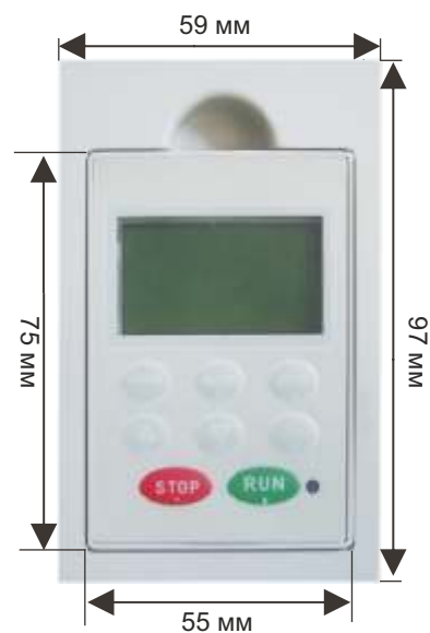
0,75 кВт - 7,5 кВт LCD панель*
