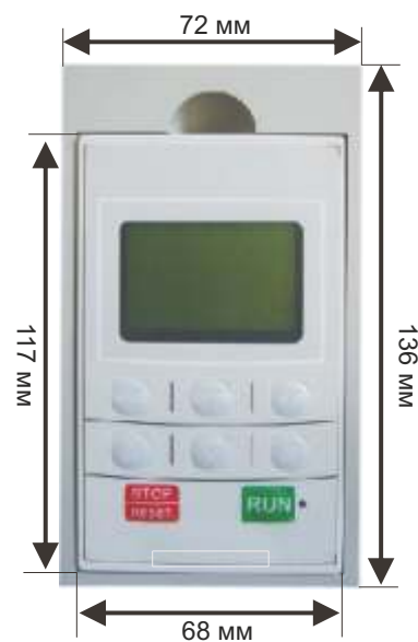
11 кВт - 630 кВт LCD панель*
